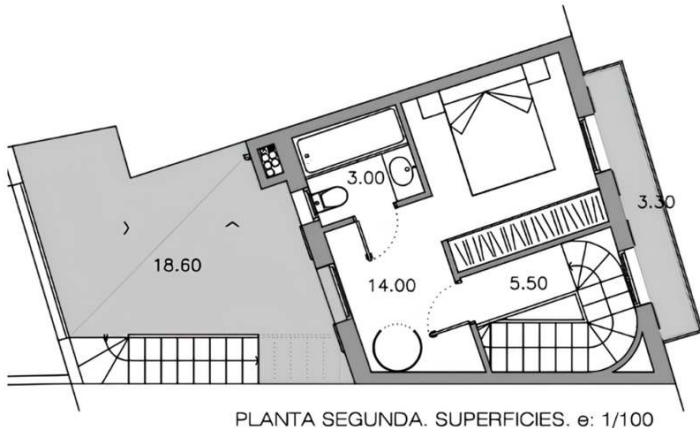
PLANTA SEGUNDA. SUPERFICIES. e: 1/100
