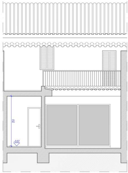
ESTADO REFORMADO - FACHADA POSTERIOR
