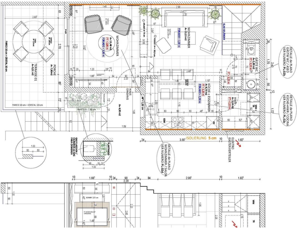
GRUNDRISSE ERDGESCHOSS / BAJA UMBAU CASA 3 - 3
