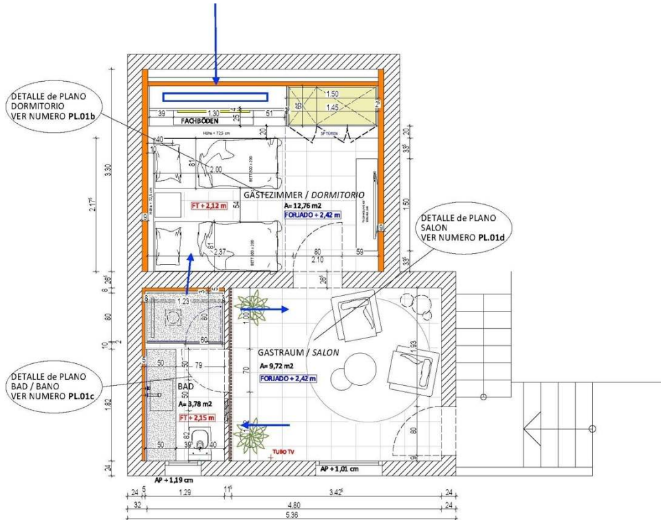
GRUNDRISS UMBAU UNTERGESCHOSS / SOTANO
