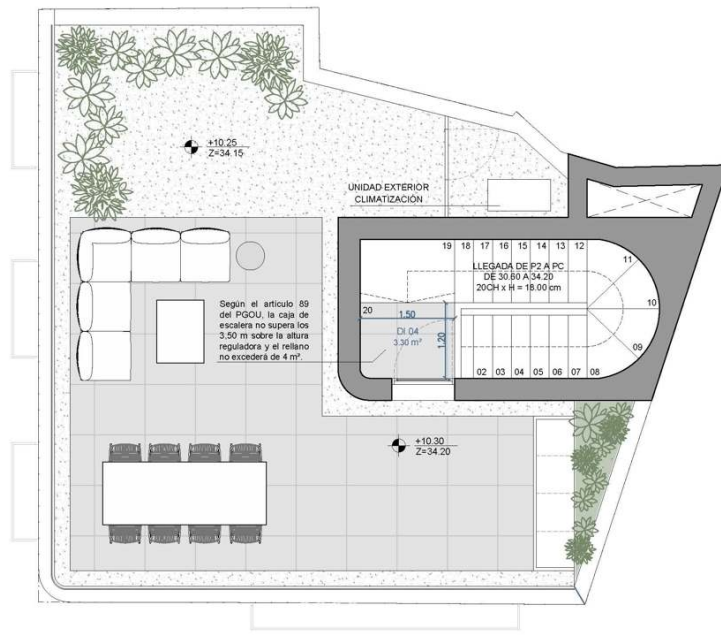
PLANTA AZOTEA 01. ESCALA 1/50
