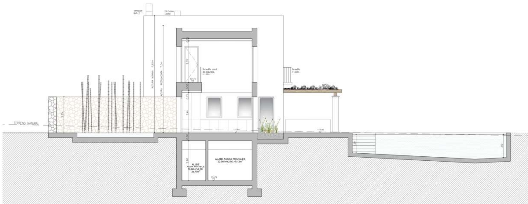
SECCIÓN C-C"
