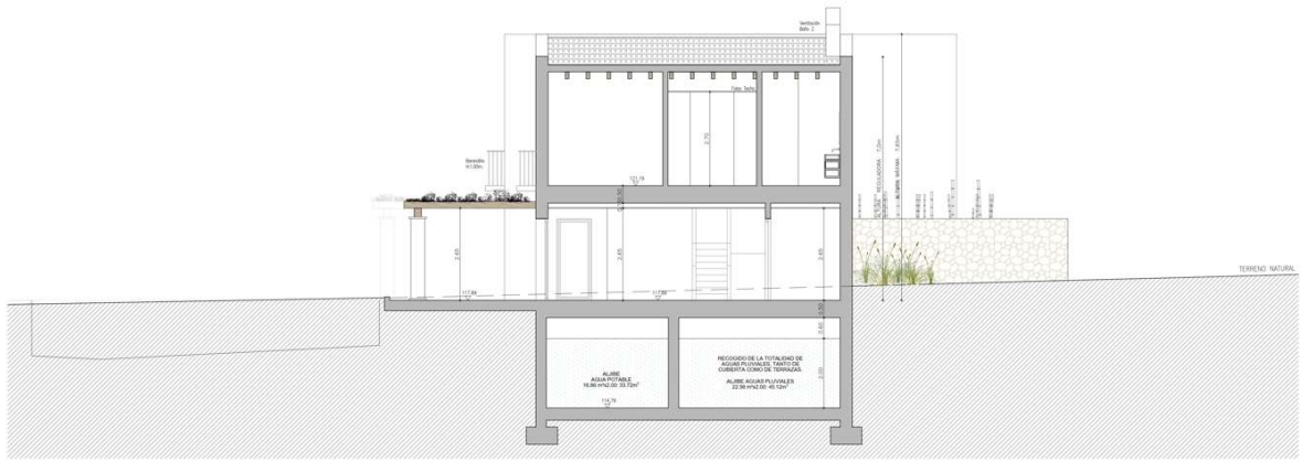
SECCIÓN B-B"
