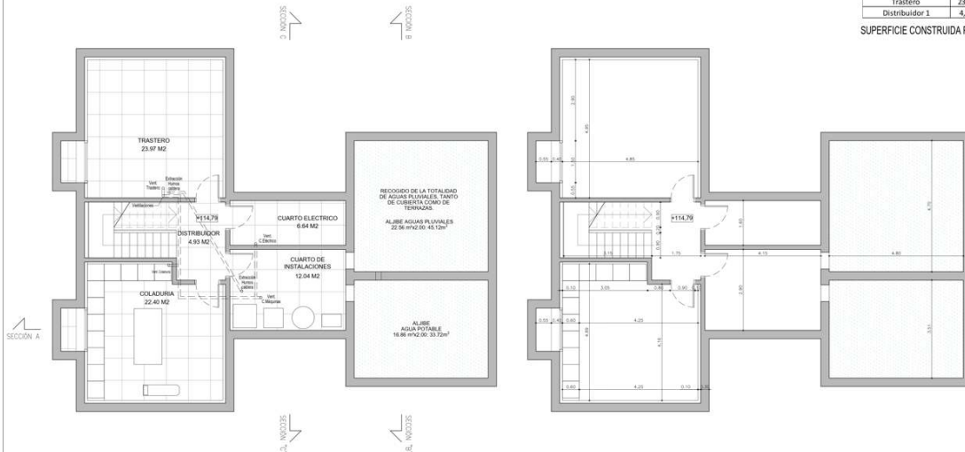
PLANTA SÓTANO SUPERFICIES ÚTILES Y MOBILIARIO.
