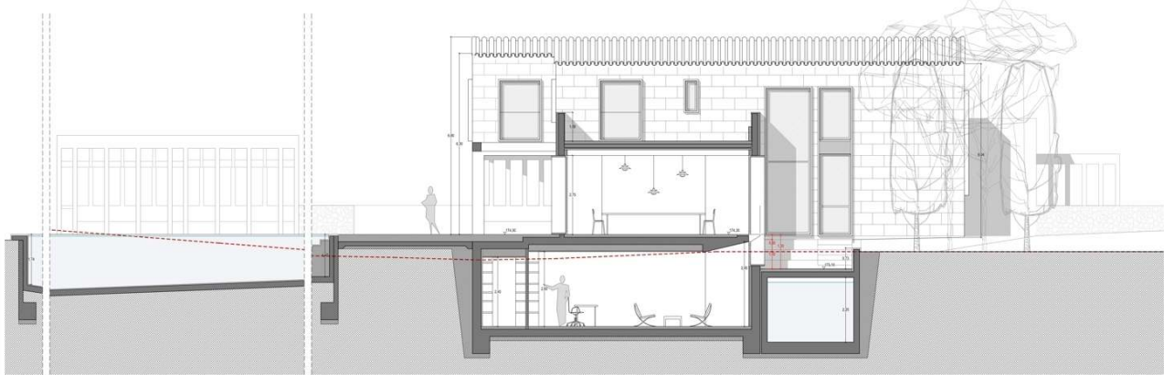
SECCION TRANSVERSAL 315 A 110
