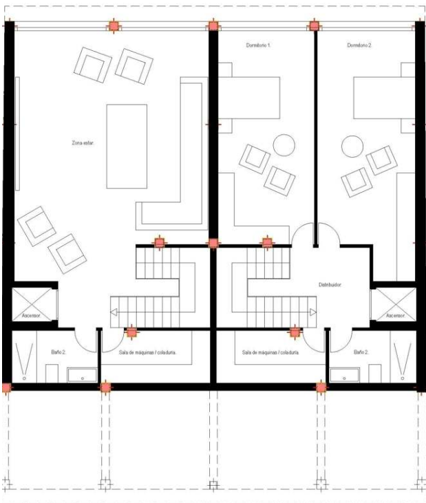
PLANTA -1.
