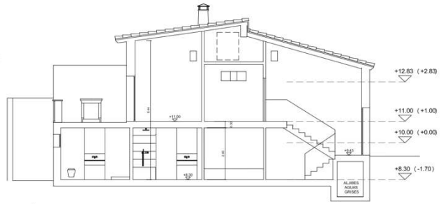
SECCIÓN 2-2'
