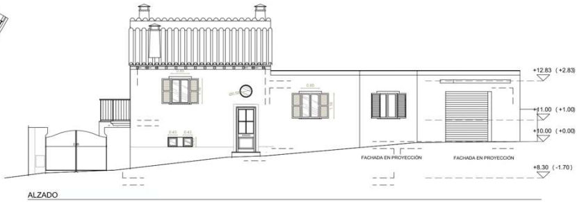
ALZADO
