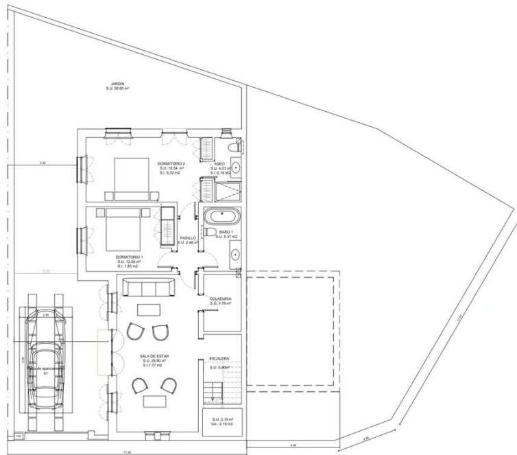
PLANTA BAJA
