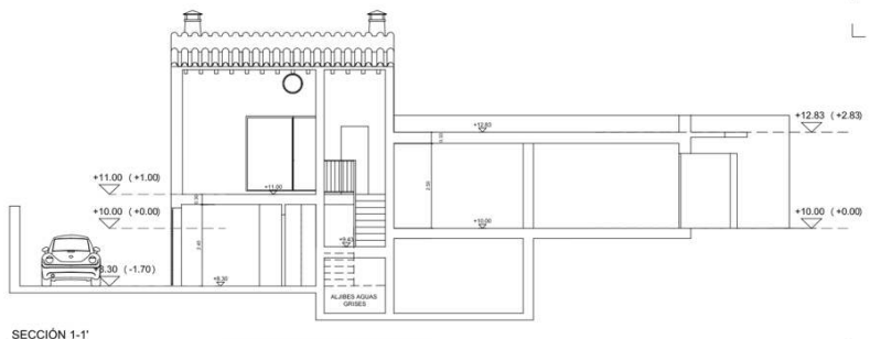
SECCIÓN 1-1'
