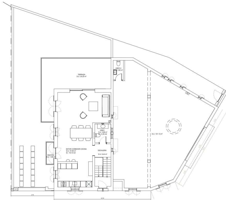
PLANTA PISO
