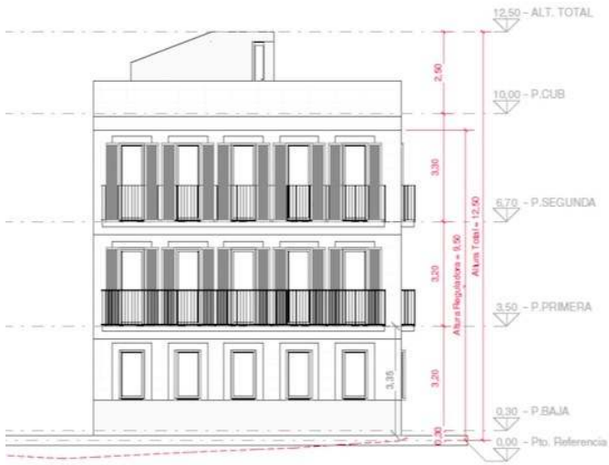
Alzado Oeste 1:100
