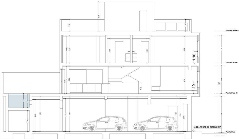
SECCION A-A' 1:50
