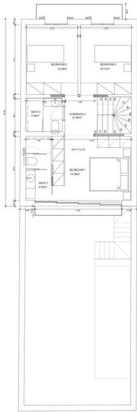
PLANTA PR10
