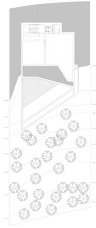
PLANTA SOTANO - IMPLANTACION EN LA PARCELA E-1029
