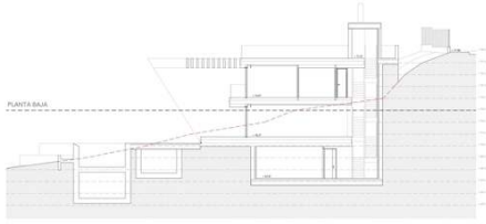
SECCION A.-B. (1/50)
