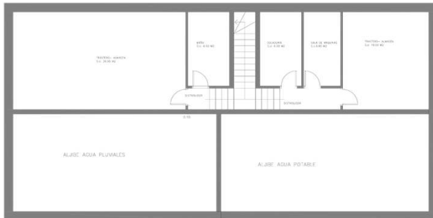
PLANTA SEGUNDO- ALJIBES Y VACIO SANITARIO
