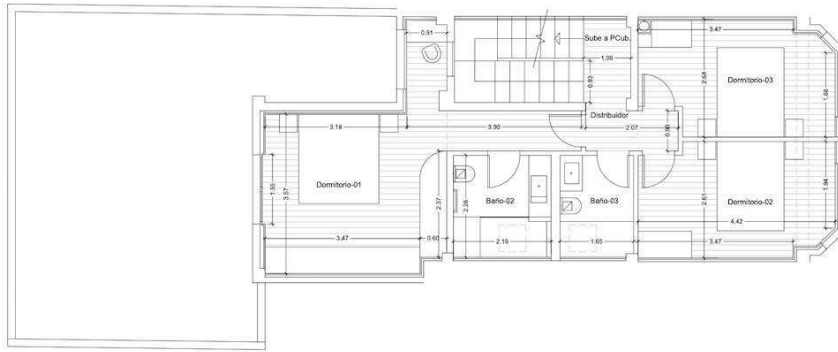
PLANTA PISO-02 Estado Reformado 1:50
