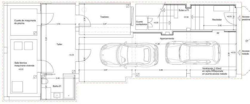
PLANTA BAJA Estado Reformado 1:50
