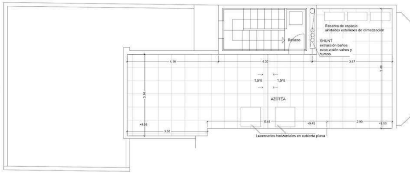
PLANTA CUBIERTA Estado Reformado 1:50
